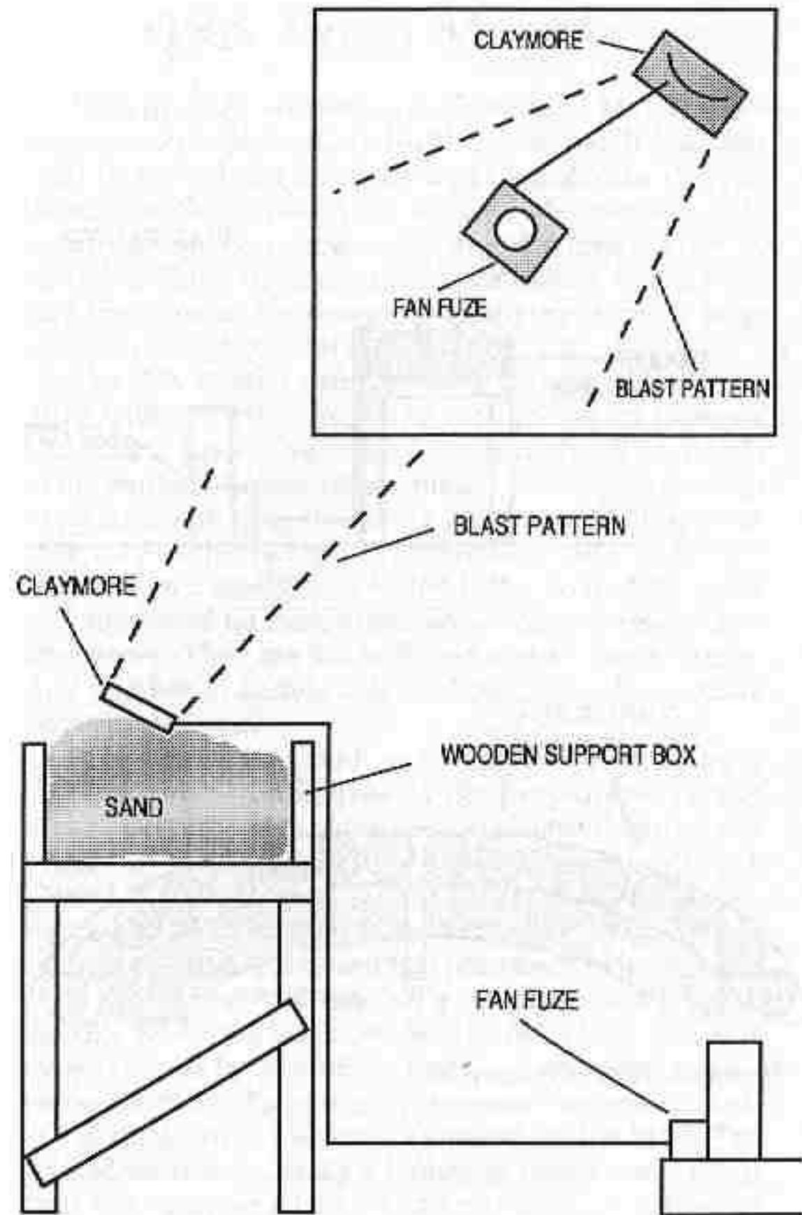
Fan fuze layout.
