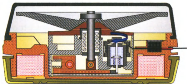
Перевод мины ПМН-4 боевое положение
