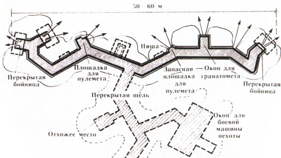
Инженерное оборудование позиции мотострелкового отделения
