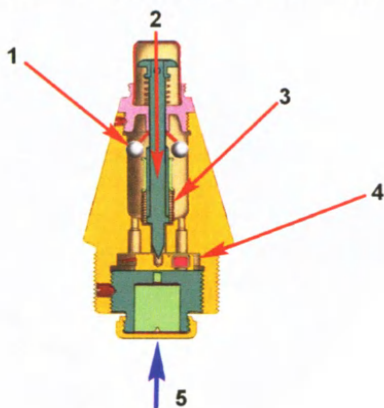
Положение основных частей осредненного головного взрывателя в момент выстрела
