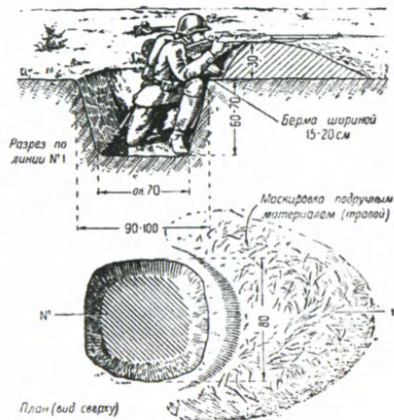
Стрелковая ячейка для ведения огня с колена Боец малой полотой отстрел ячейку и замаскирует ее за 25-30 минут
