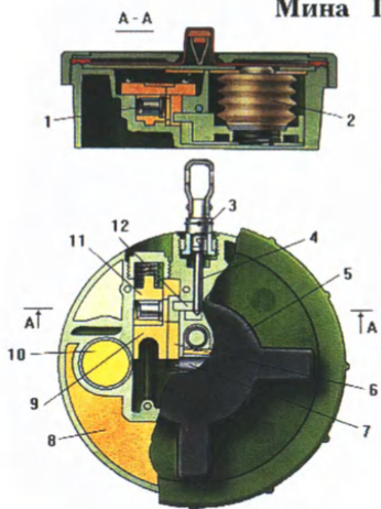
Мина ПМН-2
