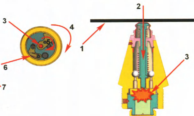
Положение основных частей осредненного головного взрывателя в момент попадания по цели
