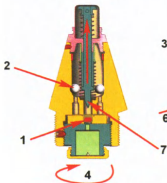
Положение основных частей осредненного головного взрывателя в полете
