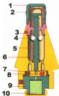
Основные части осредненного головного взрывателя
