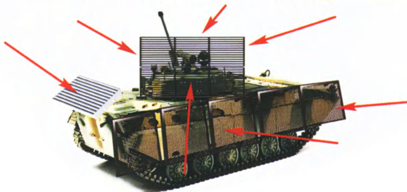
Направления вероятных ударов FPV-дронов по БМП
