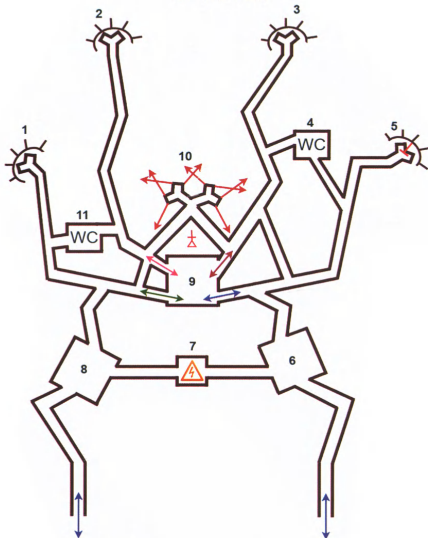
ВОП по схеме "Веер"
