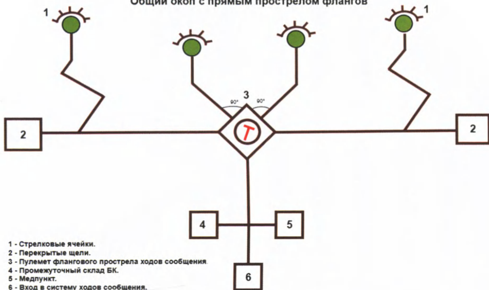
Усиление стрелковых ячеек от фланговых атак
