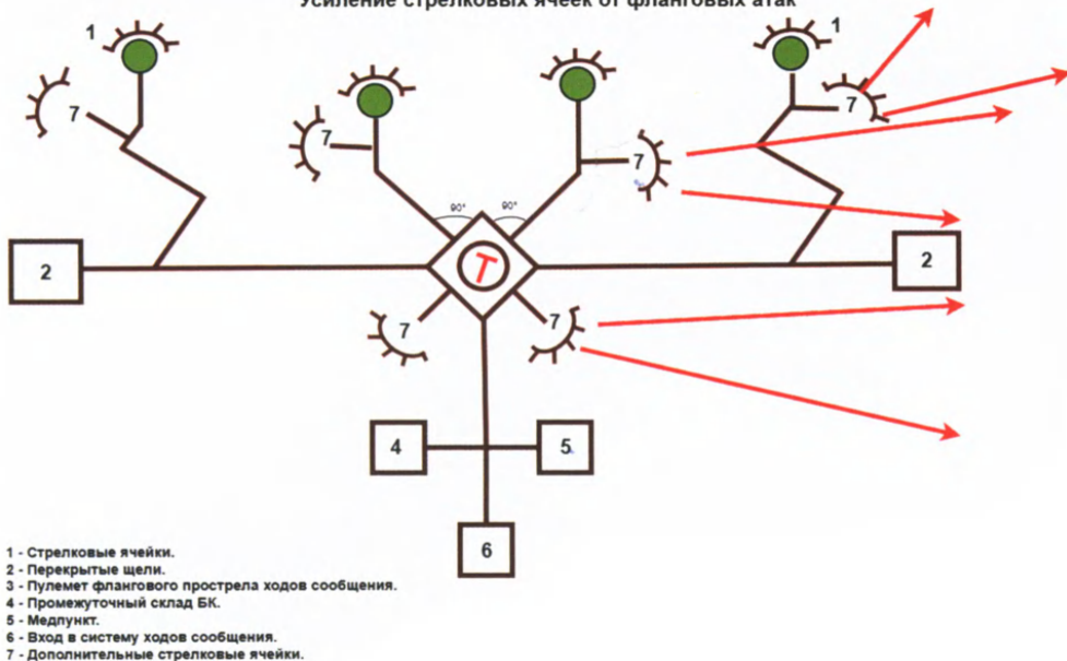
Усиление стрелковых ячеек от фланговых атак
