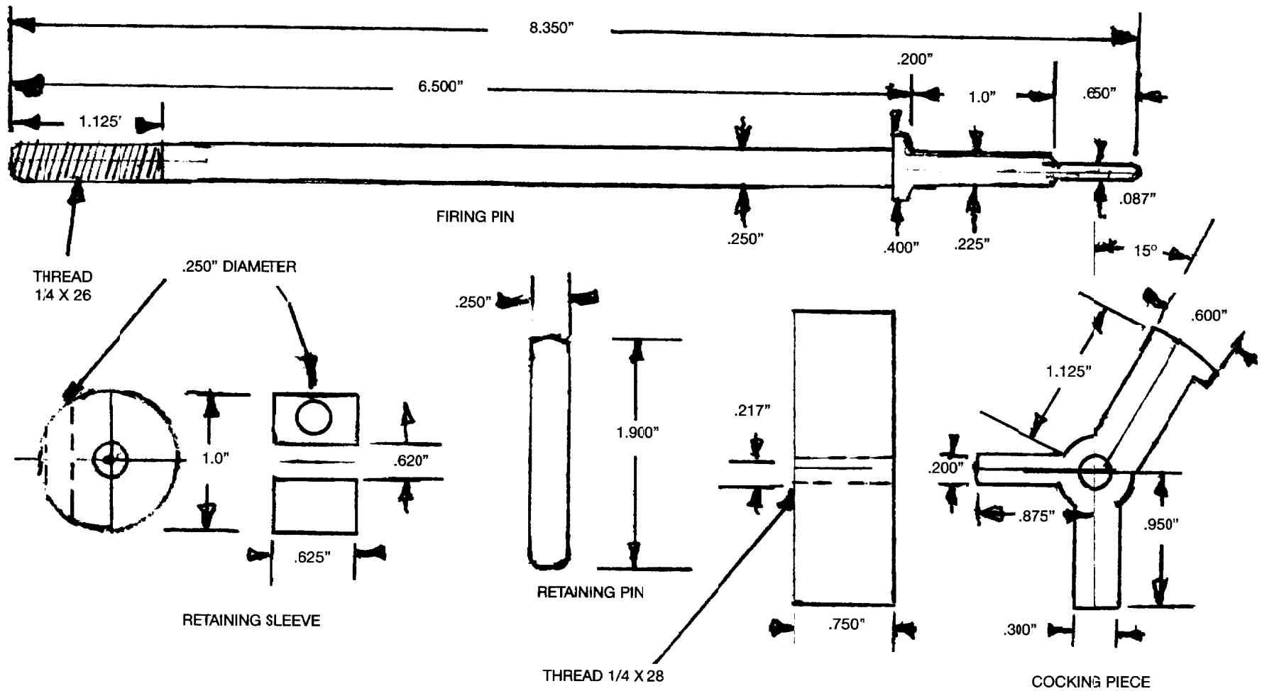
STRIKER ASSEMBLY
